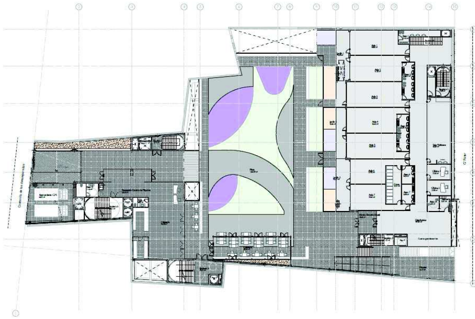
Planta Segunda
