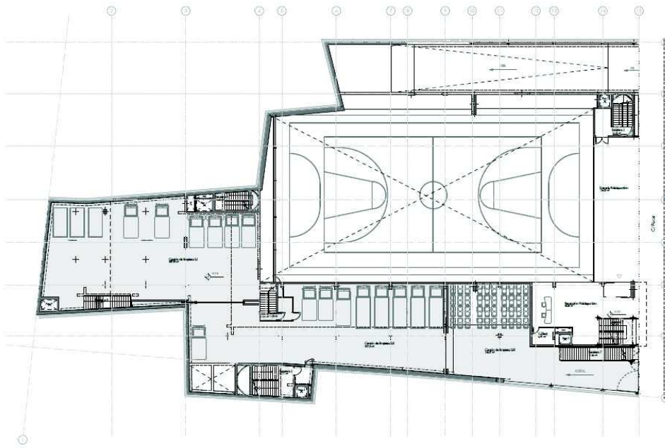
Planta Baja
