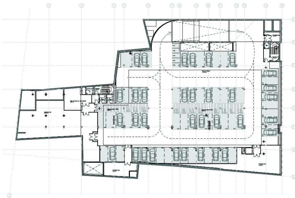
Planta Sótano -2
