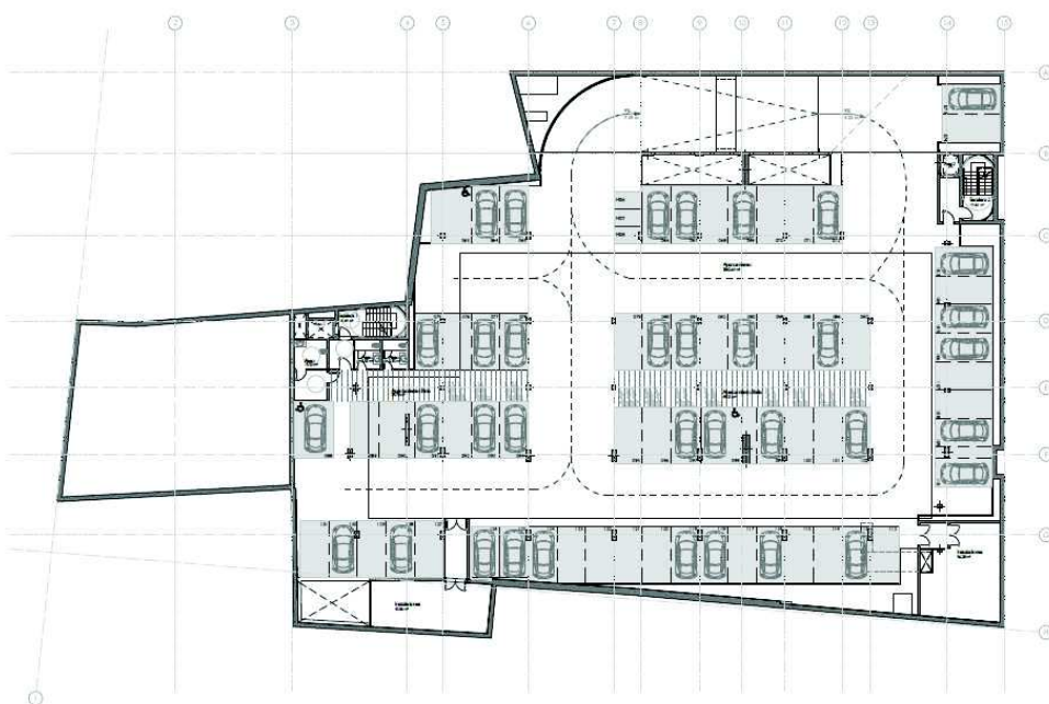
Planta Sótano -3
