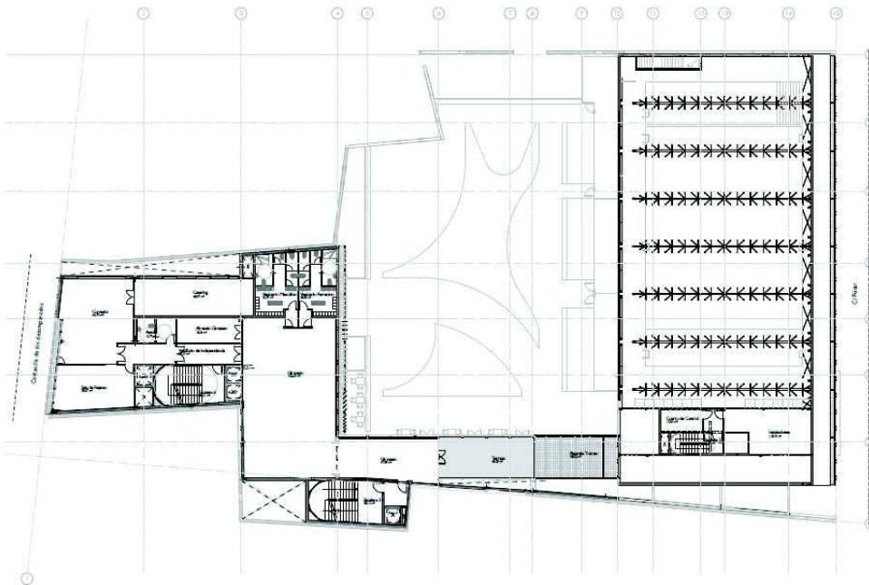
Planta Quinta
