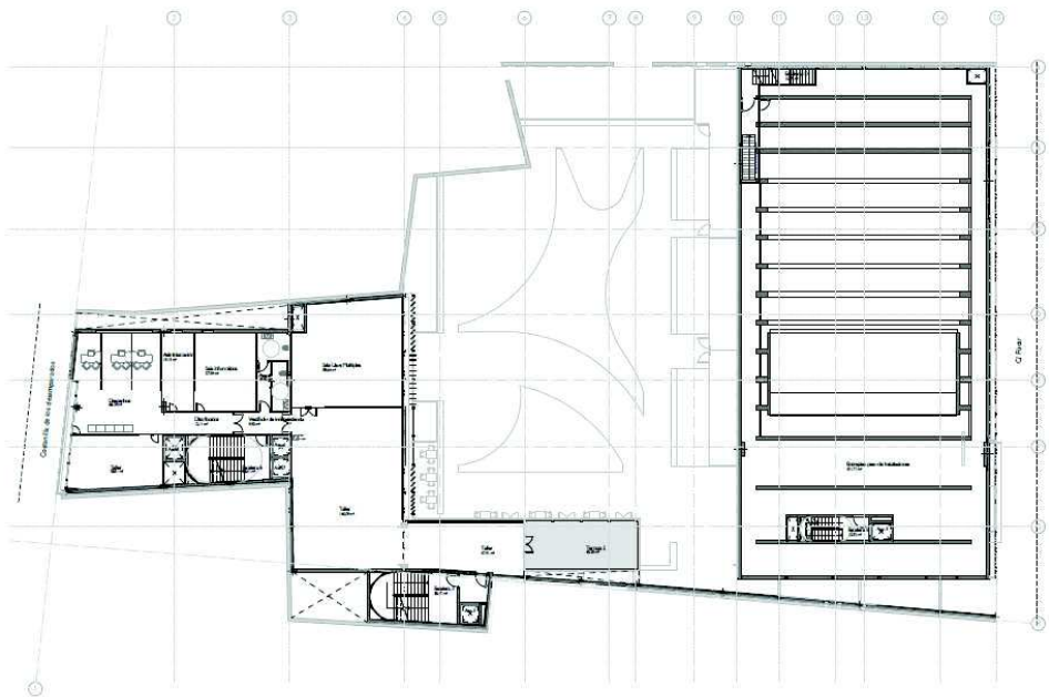
Planta Tercera
