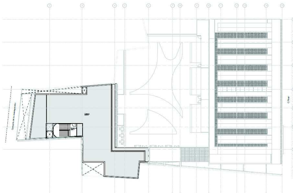
Planta Séptima
