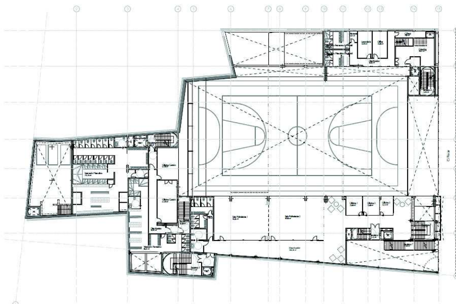
Planta Primera
