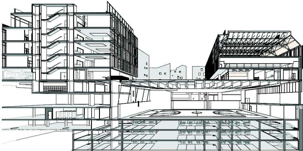
Sección fugada
